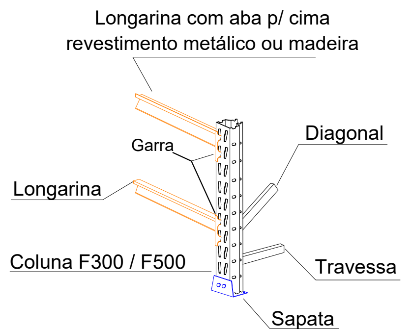
Detalhes estruturais Mini porta pallets
