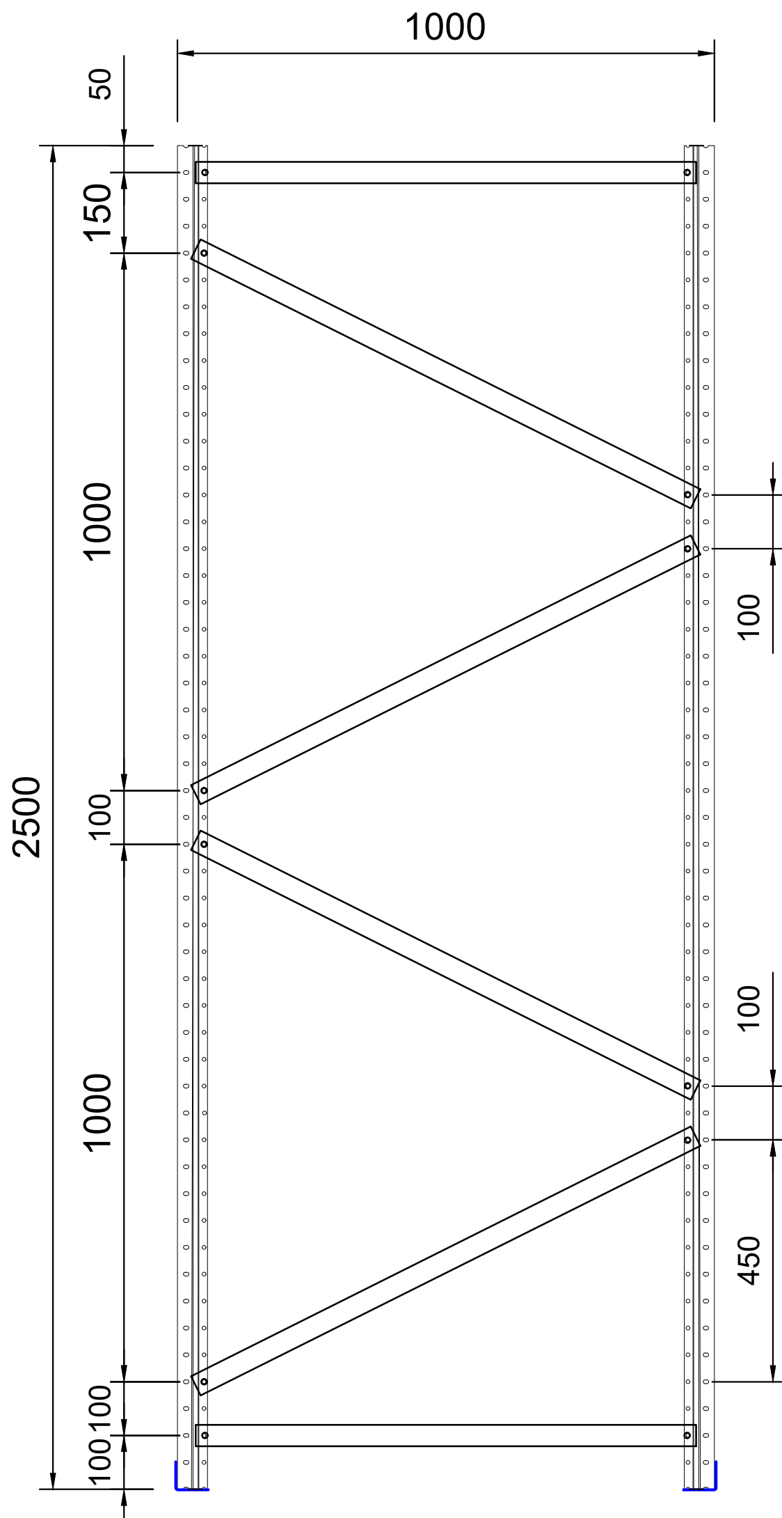
Modelo de montagem dos montantes
