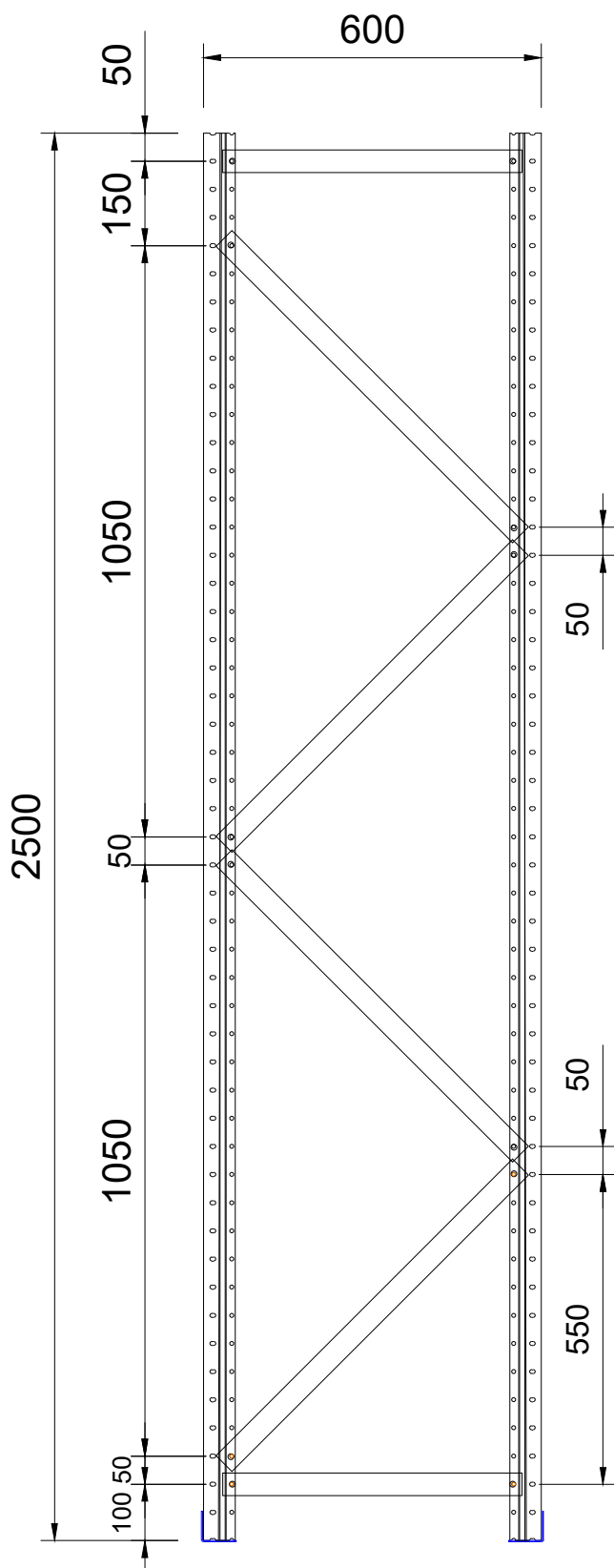
Modelo de montagem dos montantes
