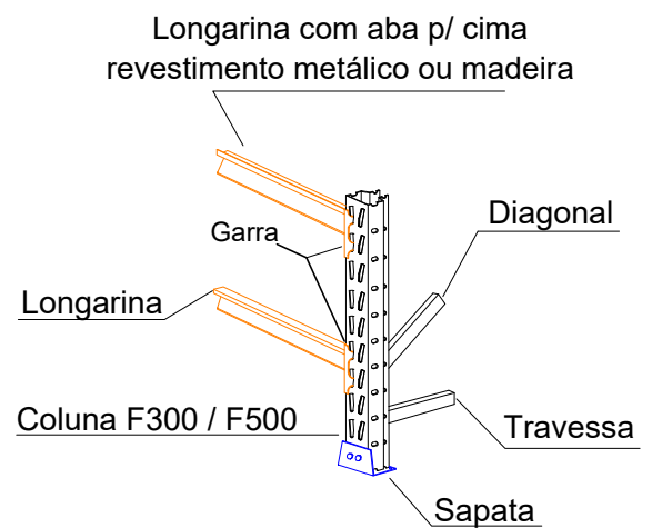
Detalhes estruturais Mini porta pallets
