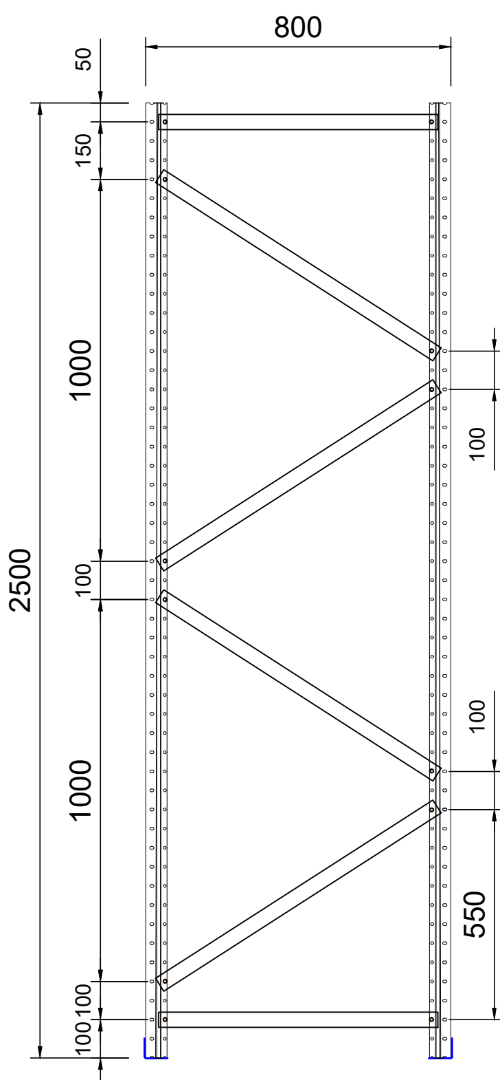
Modelo de montagem dos montantes
