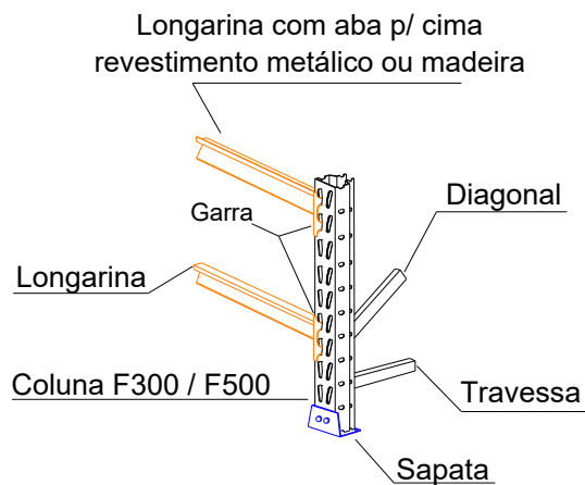
Detalhes estruturais Mini porta pallets
